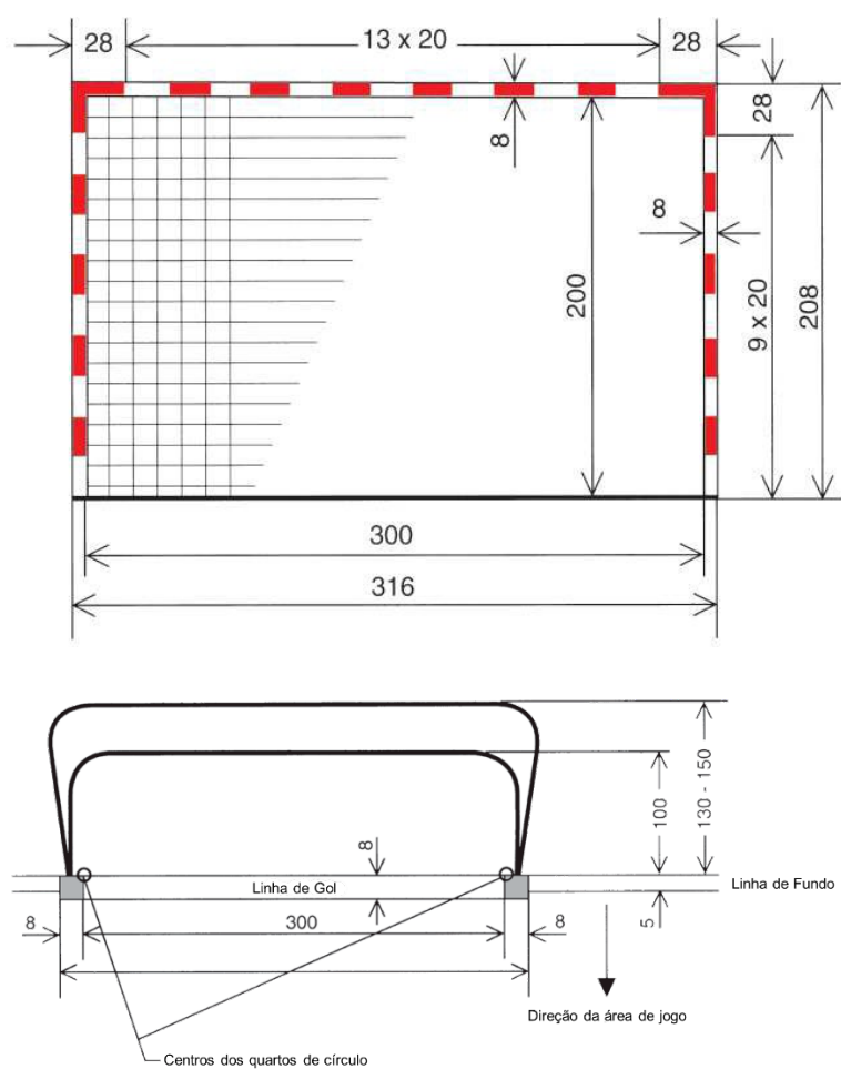
Figura 2b: A Baliza – Vista Lateral
