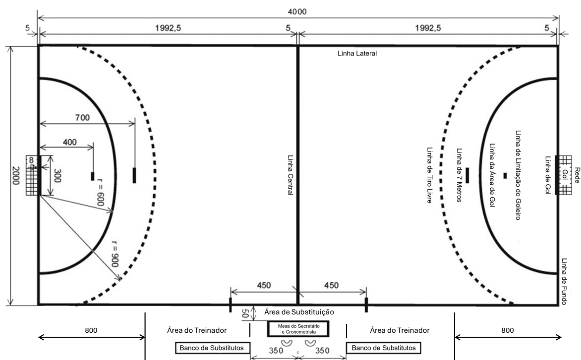
Figura 1a: A Quadra de Jogo – somente com a Linha Central Dimensões indicadas em cm.
