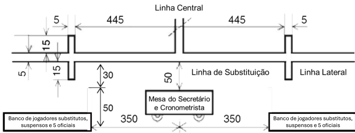
Figura 3: Linhas e Área de Substituição
